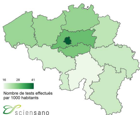
Nombre de tests effectués par province, par 1000 habitants entre le 18/08/21 et le 24/08/21
