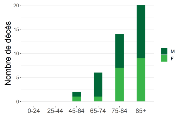
Distribution du nombre de décès COVID-19 par âge et sexe (18/08/21-24/08/21)
