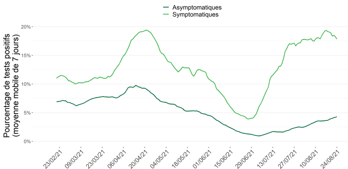
Taux de positivité en fonction de la présence ou non de symptômes (moyenne mobile sur 7 jours), en pourcentage, pour la période du 15/02/21 au 24 août 2021
