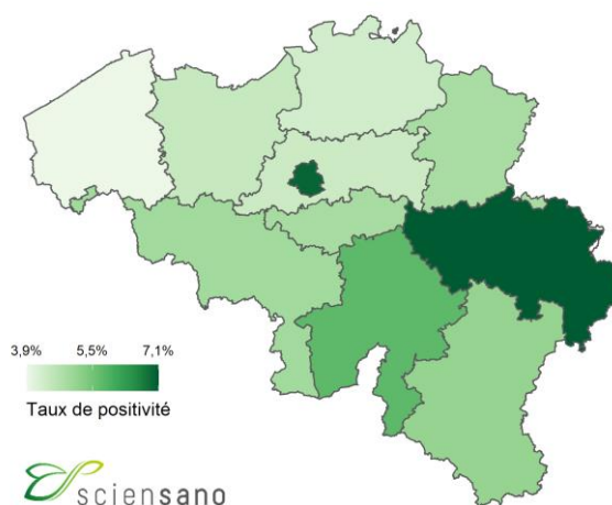
Taux de positivité par province entre le 18/08/21 et le 24/08/21
