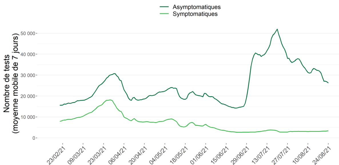
Tests effectués en fonction de la présence ou non de symptômes (moyenne mobile sur 7 jours), pour la période du 15/02/21 au 24 août 2021
