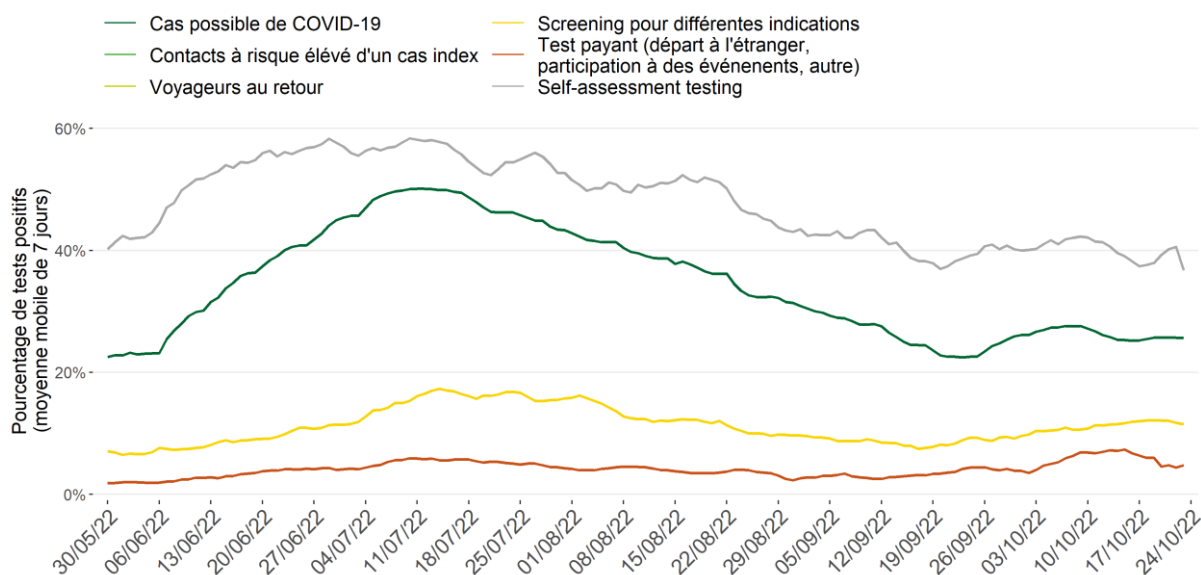
Évolution du taux de positivité par indication de test pour les prescriptions disponibles, pour la période du 30/05/22 au 23/10/22
