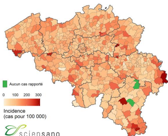
Distribution des cas confirmés par 100 000 habitants entre le 22/10/22 et le 04/11/22
