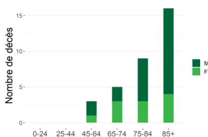
Distribution du nombre de décès COVID-19 par âge et sexe (29/10/22-04/11/22)
