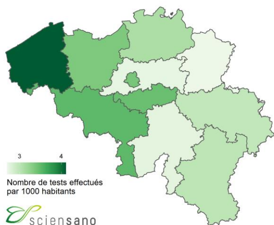
Nombre de tests effectués par province, par 1000 habitants entre le 29/10/22 et le 04/11/22
