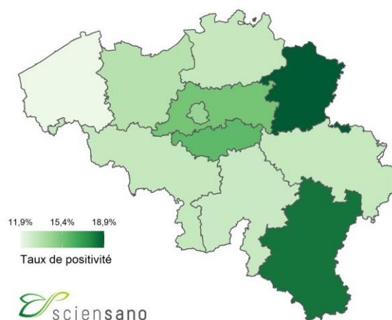
Taux de positivité par province entre le 29/10/22 et le 04/11/22
